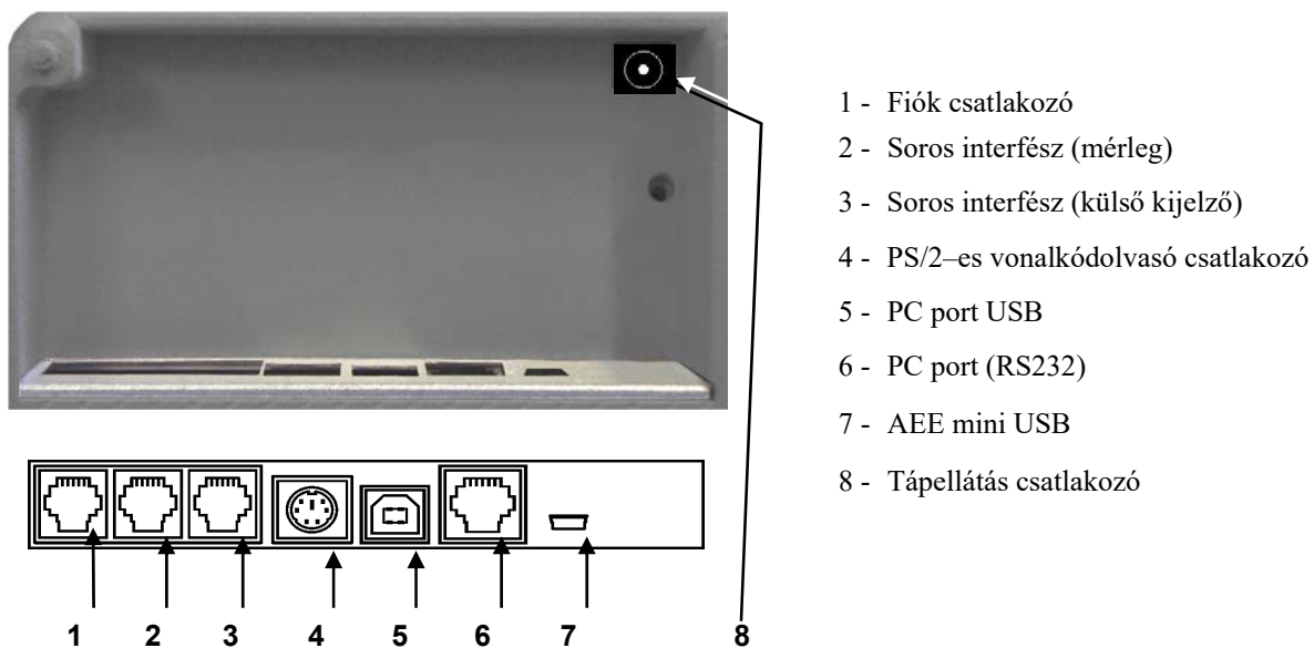
2. ábra - Csatlakozók a pénztárgép alján
