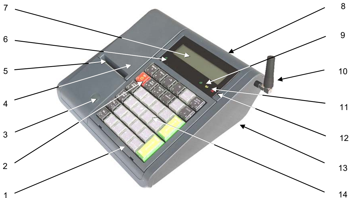
1. ábra - Pénztárgép elől nézet.
